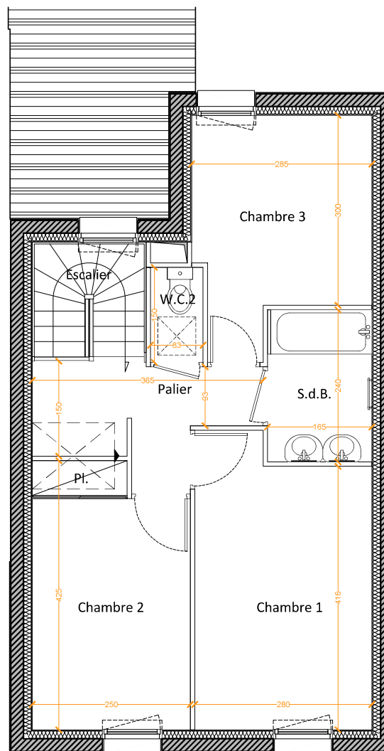
plan de l'étage
